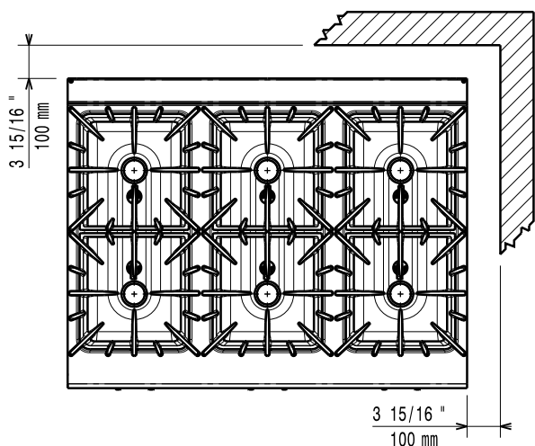
Felülnézet
